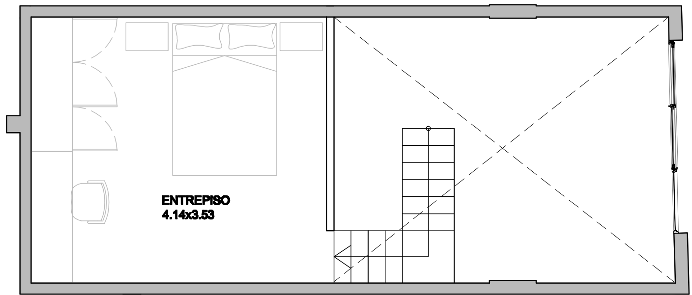
PLANTA NIVEL SUPERIOR
